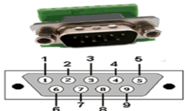
Figura 11: Modelo de Porta Serial de 9 pinos.
