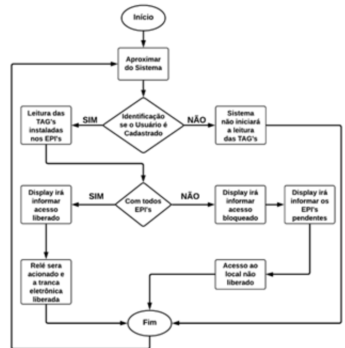
Figura 22: Fluxograma de funcionamento e condições do sistema desenvolvido.
