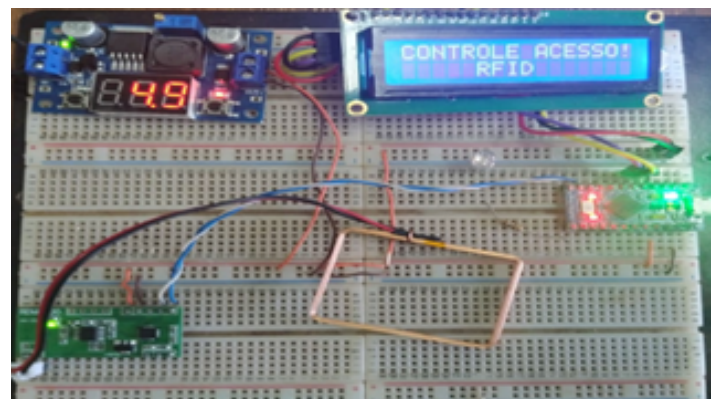
Figura 21: Ligações dos dispositivos do sistema.
