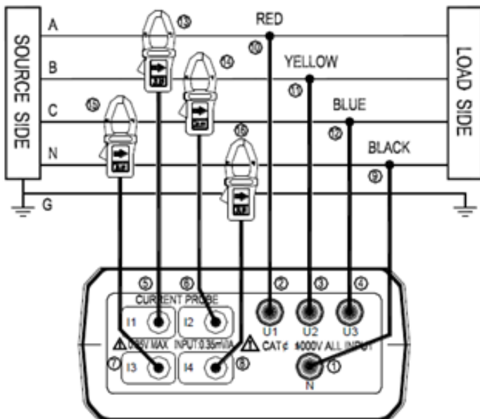
Figura 1: Diagrama de conexão do analisador aos cabos.
