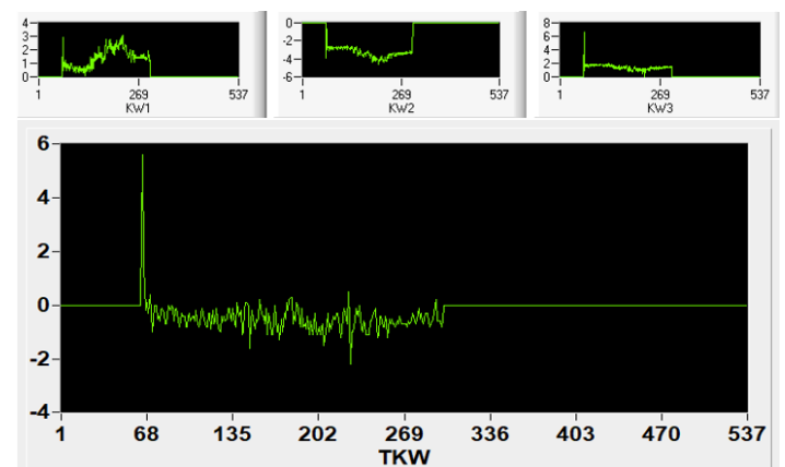
Figura 9: Medição do Fator de Potência.
