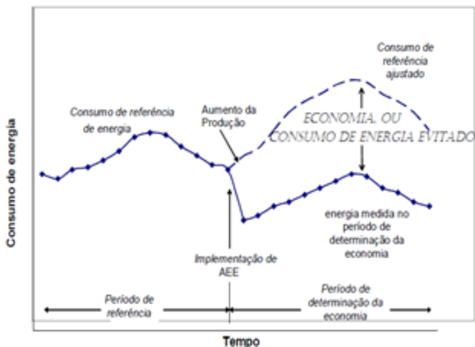
Figura 19: Histórico de Energia.
