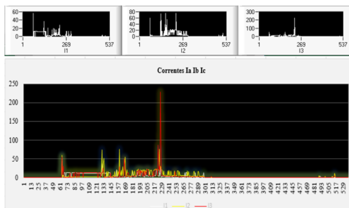
Figura 5: Correntes I1, I2 e I3.
