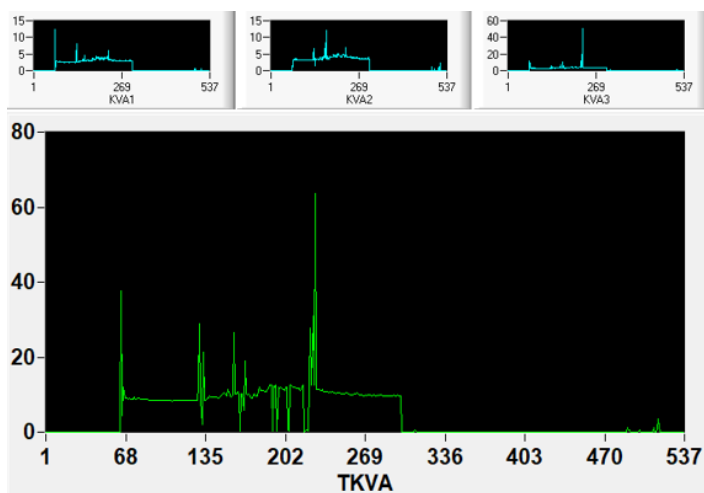
Figura 11: Medição do Fator de Potência.
