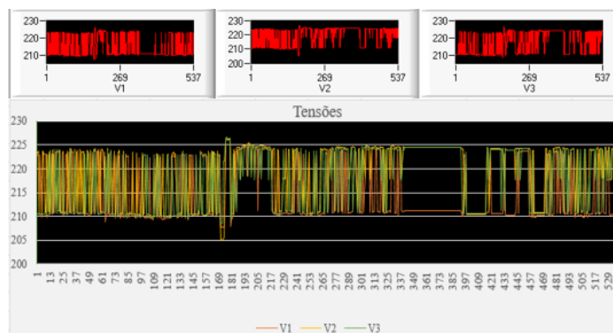
Figura 4: Tensões V1, V2 e V3.
