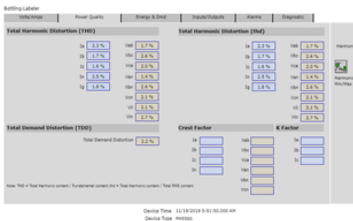
Figura 15: Tela do Sistema - Power Monitoring Expert.
