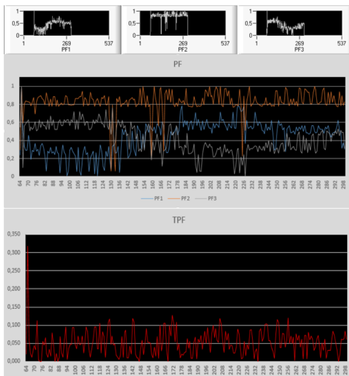
Figura 6: Medição do Fator de Potência.
